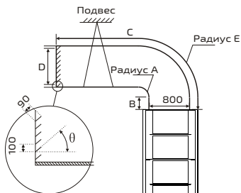
Размеры выходной решетки (приобретается отдельно)
