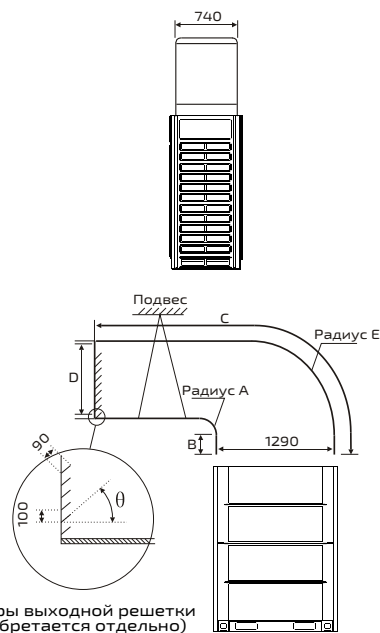
Размеры выходной решетки (приобретается отдельно)
